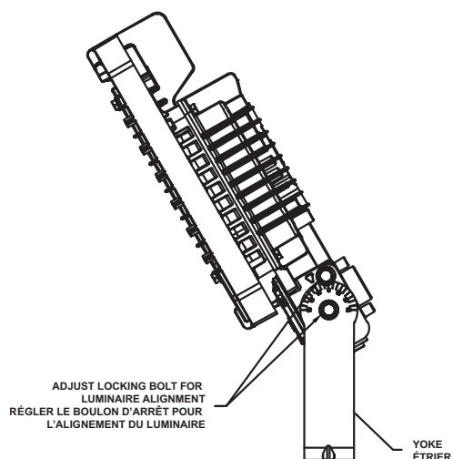
Figure 3: Adjusting the Luminaire with Yoke | Réglage du luminaire avec étrier
